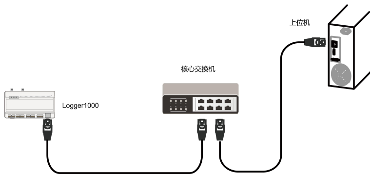
图 6-2 与光伏系统后台连接示意图
