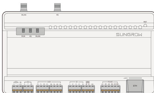
图 6-1 接线区域
