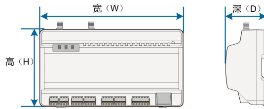
图 3-2 产品尺寸
