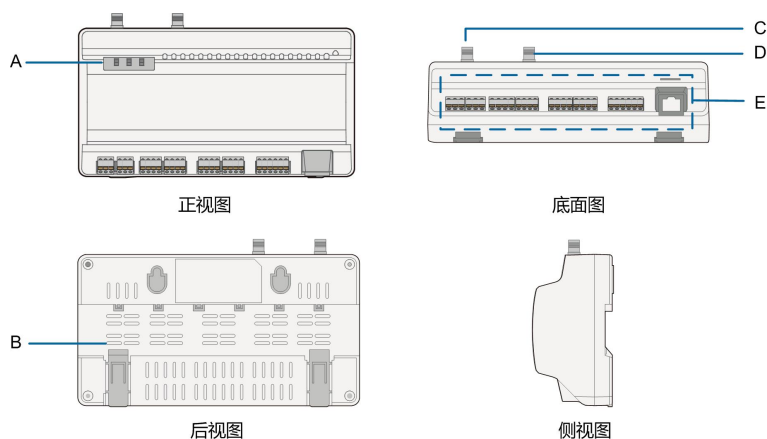
图 3-1 产品外观
