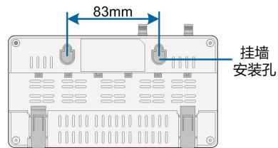
图 5-1 挂墙安装孔尺寸
