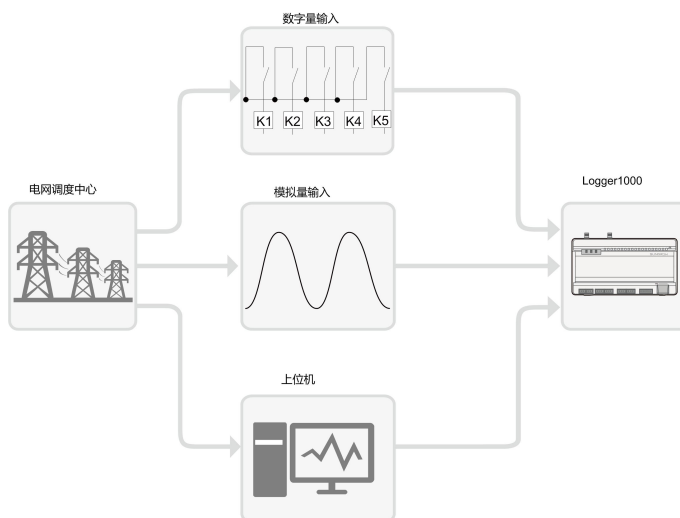
图 9-1 功率控制功能整体架构
