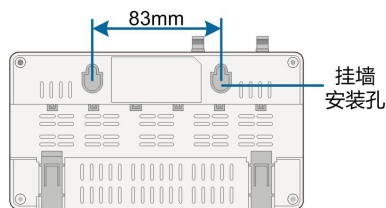
图 4-1 挂墙安装孔尺寸
