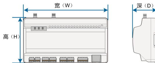
图 2-2 产品尺寸
