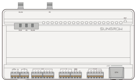
图 5-1 接线区域
