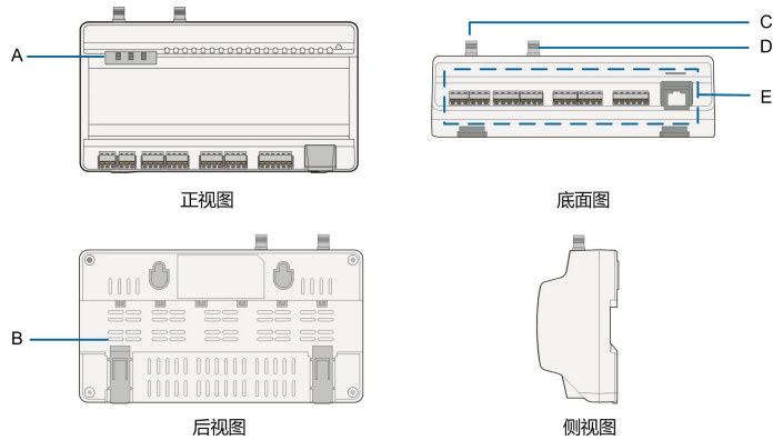
图 2-1 产品外观
