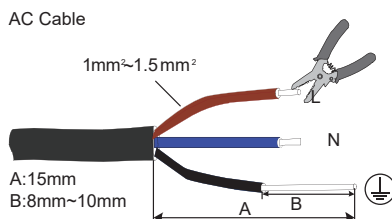
AC Cable
