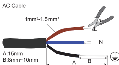
AC Cable
