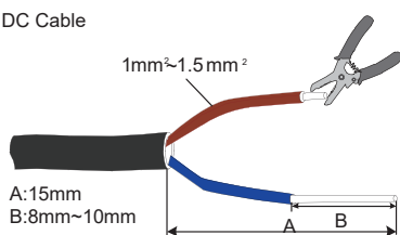
DC Cable
