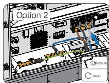
7-2 AC and equipotential bonding scheme 2
